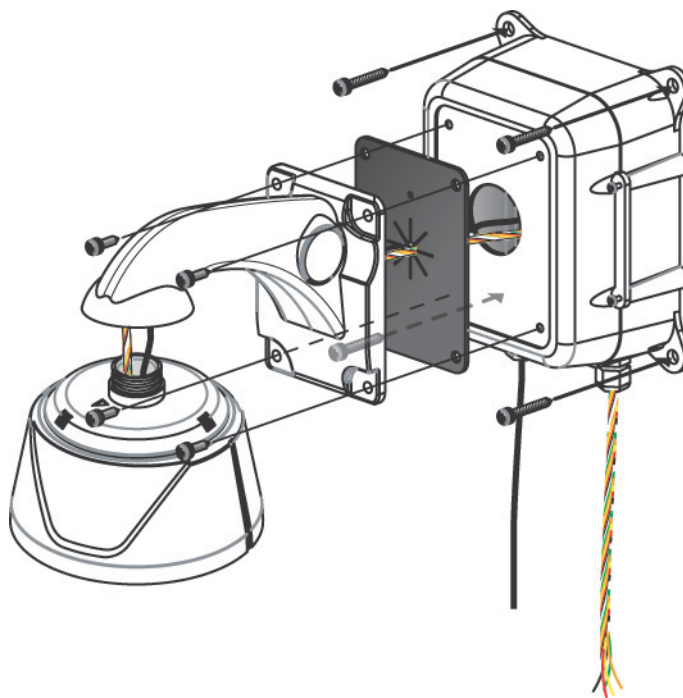
Монтаж распределительной коробки купольной камеры
